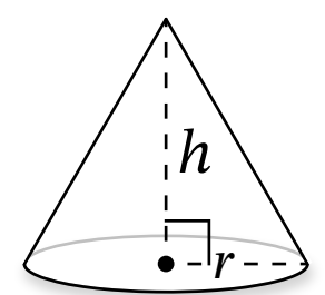
Cone
